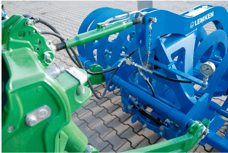
Bild 3: Neuer LEMKEN Frontpacker VarioPack
